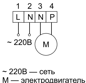
Схема подключения
